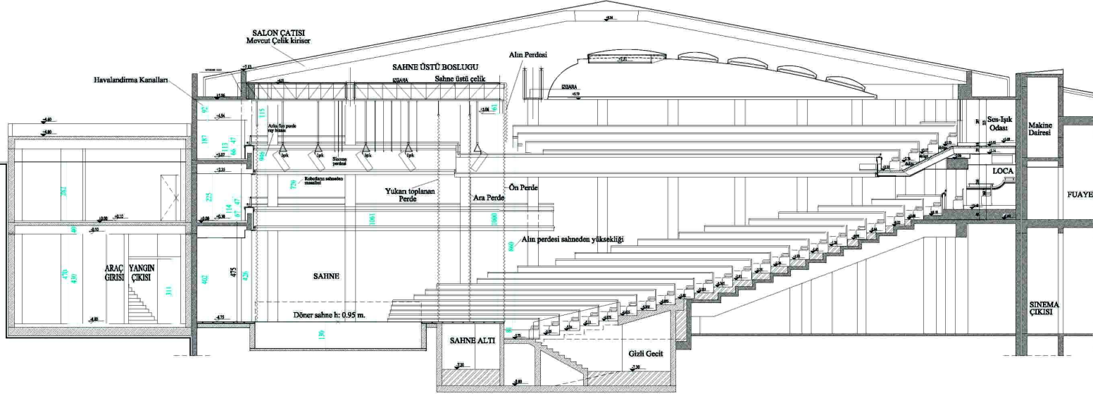
SALON KESİTİ
